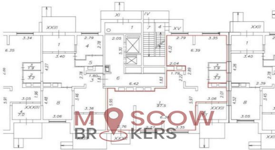
Масштаб 1:200
